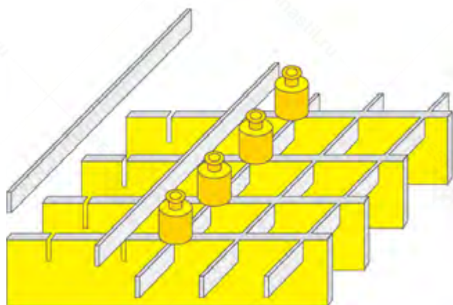
Рис. 1. Изготовление прессованного решетчатого настила (P). Запрессовка покровных полос в несущие полосы под давлением в 5000 кН (около 500 тонн).
